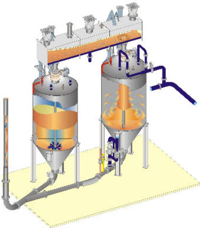
Transporte pneumático em fase densa/ Pneumatic conveying dense phase
