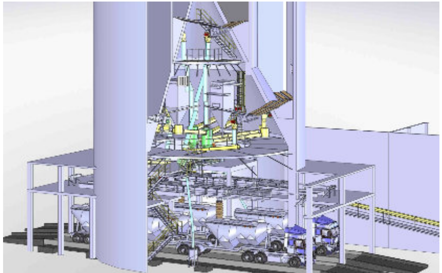
Silo de cone invertido / Inverted cone silo
