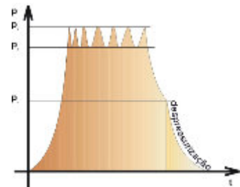
Pressões durante transporte por fase densa / Dense phase conveying pressure behavior
